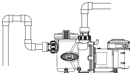
Figura 3 - INSTALACIÓN INCORRECTA
