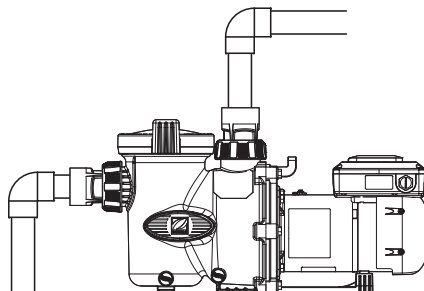
FIGURA 2 - INSTALLAZIONE CORRETTA
