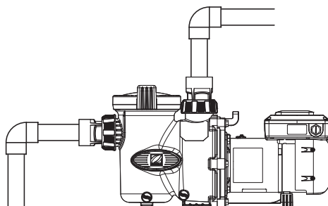
FIGURA 2 - INSTALLAZIONE CORRETTA
