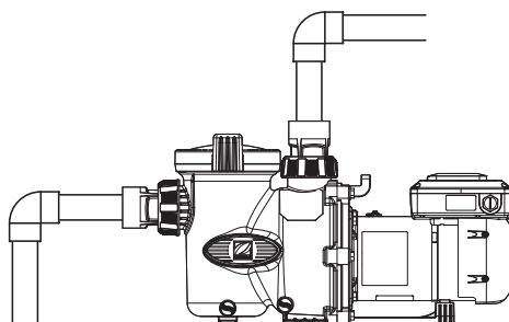
FIGURA 2 - INSTALAÇÃO CORRETA
