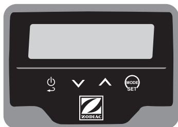
FIGURA 8 - CONTROLLI IN MODALITÀ DI FUNZIONAMENTO NORMALE
