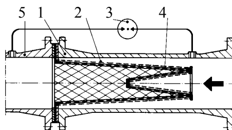
(Filter für Ansaugleitung)
